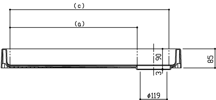
断面A-A
